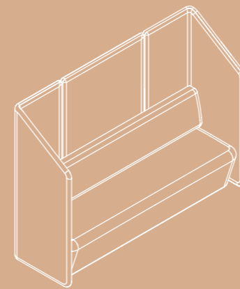
W 2160 x D 720 x H 1600 mm
