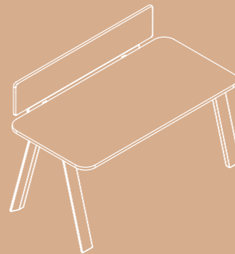
W 1200 / 1400 / 1600 / 1800 x D 821 x H 740/1070 mm
